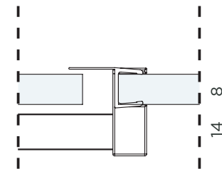
GIUNZIONE PORTA / VETRO FISSO JOINT DOOR / FIXED GLASS
