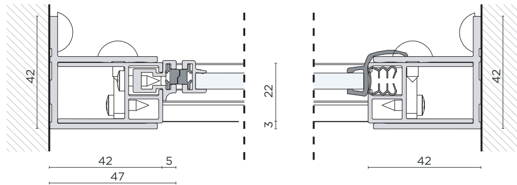
PROFILO A PARETE CON BATTUTA PORTA WALL PROFILE WITH DOOR STOP
